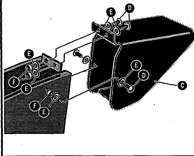
FIG. 4-ASSY
